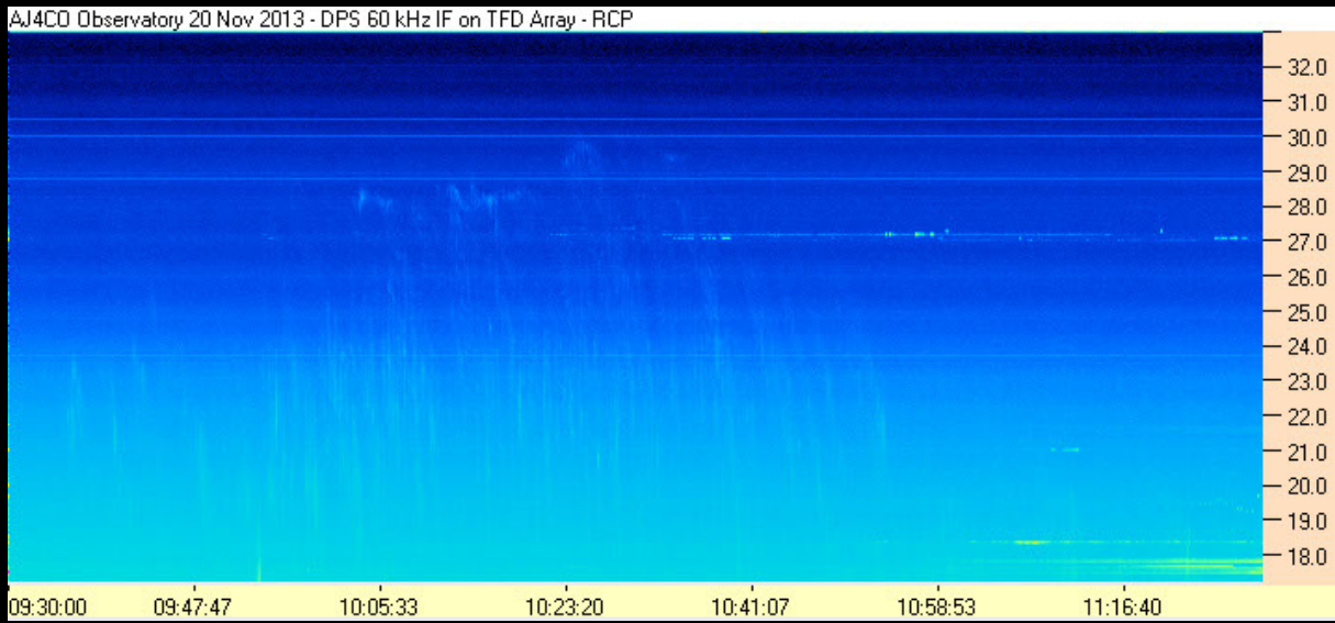
Io-A 131120093000AJ4CO DPS.PNG
